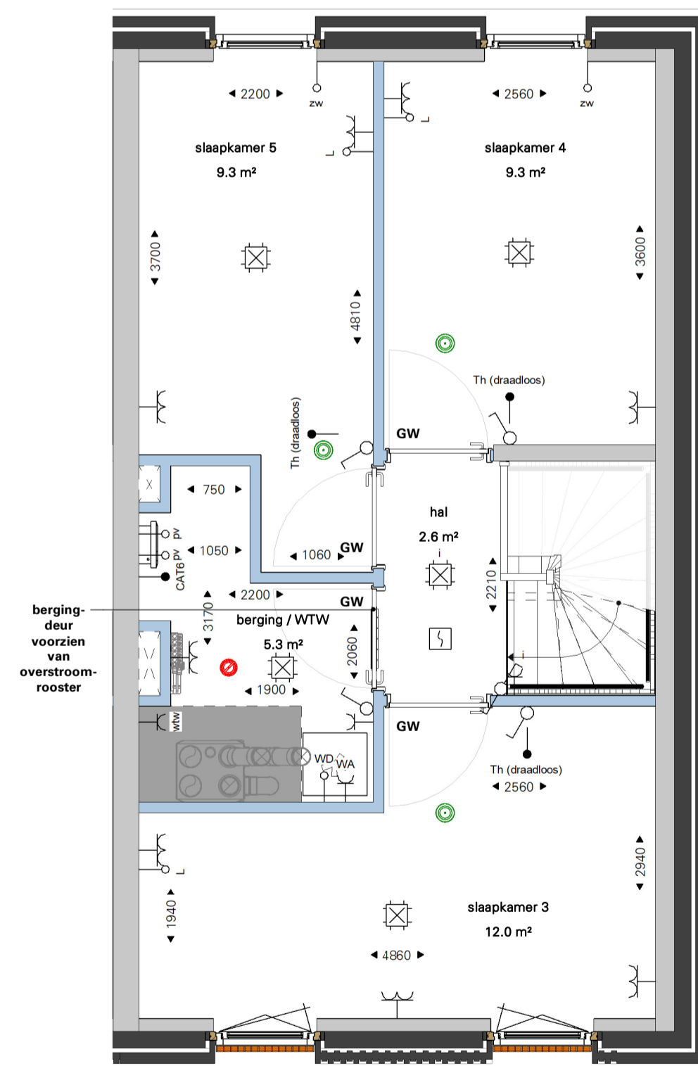
derde verdieping
