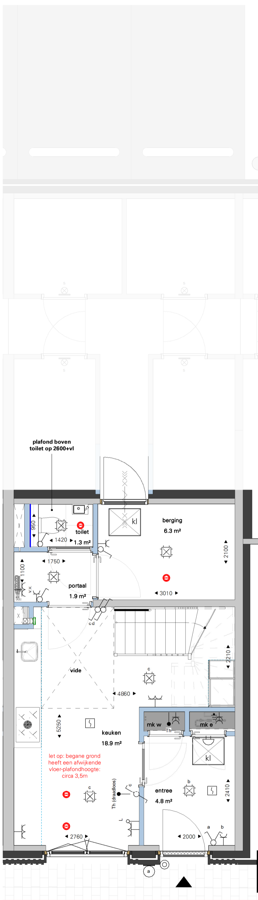
begane grond
